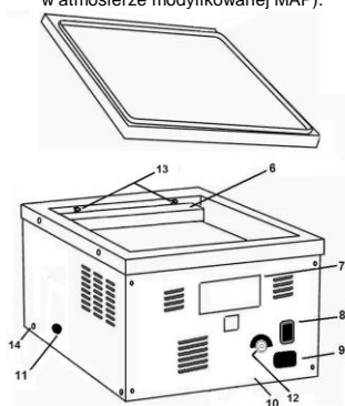
Widok z tyłu – modele CVP350 i CVP450
