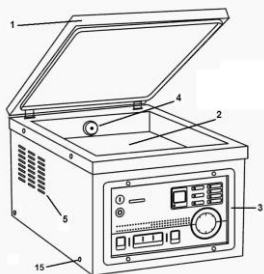
Widok z przodu – Modele CVP260/300/350/450
